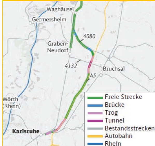
Vorzugsvariante R4, Quelle: DB
